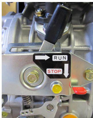
Ручка-переключатель «RUN-STOP» в положении «РАБОТА»
