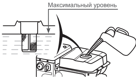
Рис. 5 Максимальный уровень топлива в топливном баке
