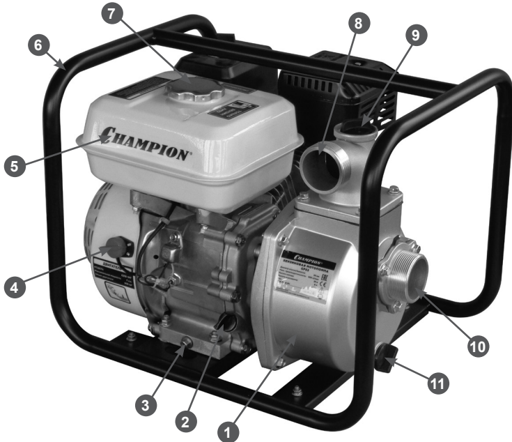
Рис. 2 Основные узлы и органы управления (общий вид)
