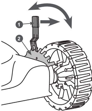
Рис. 15 Регулировка высоты скашивания
