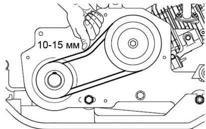
Рис. 20 Проверка натяжения ремня привода вибратора
